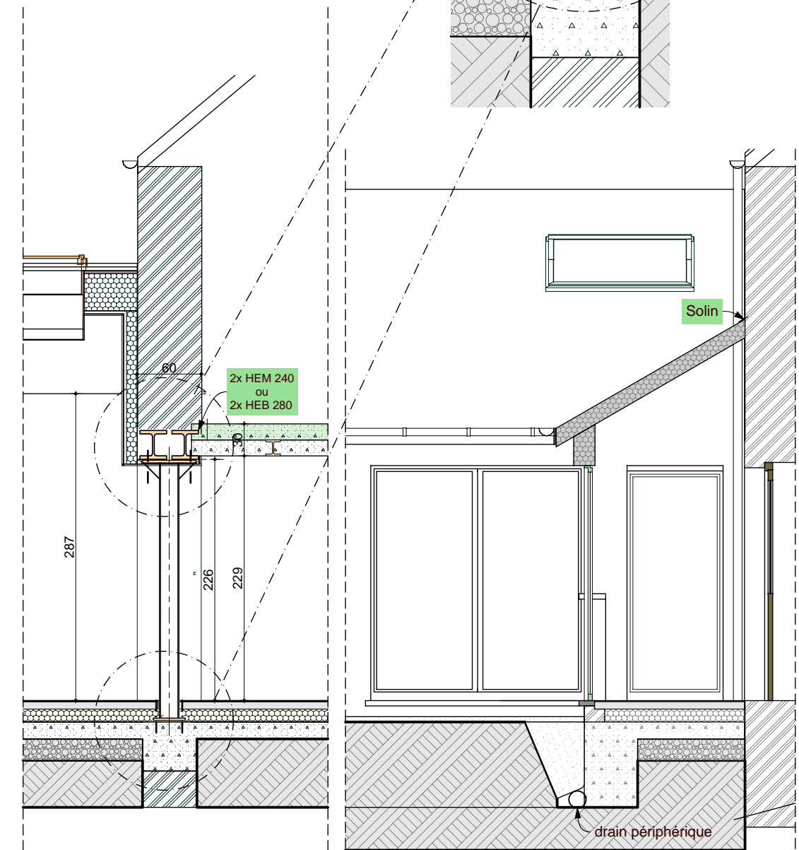
COUPE EE
