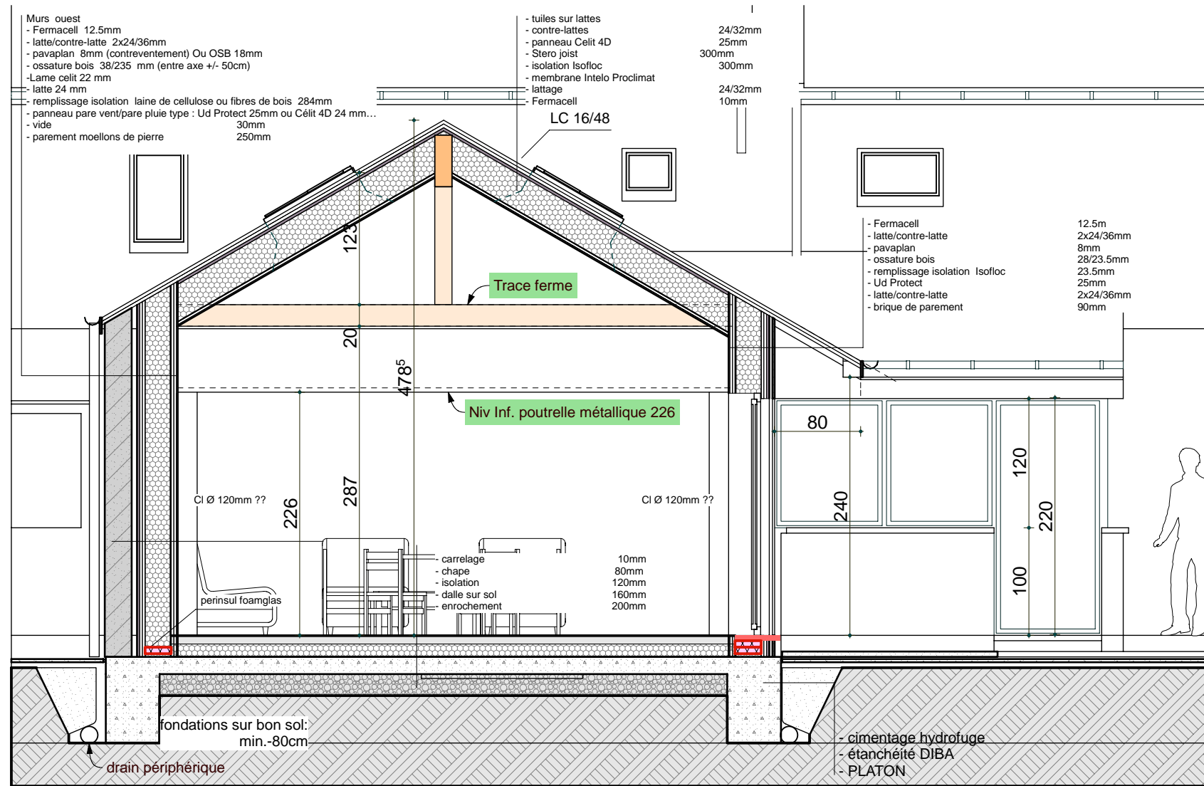
COUPE BB
