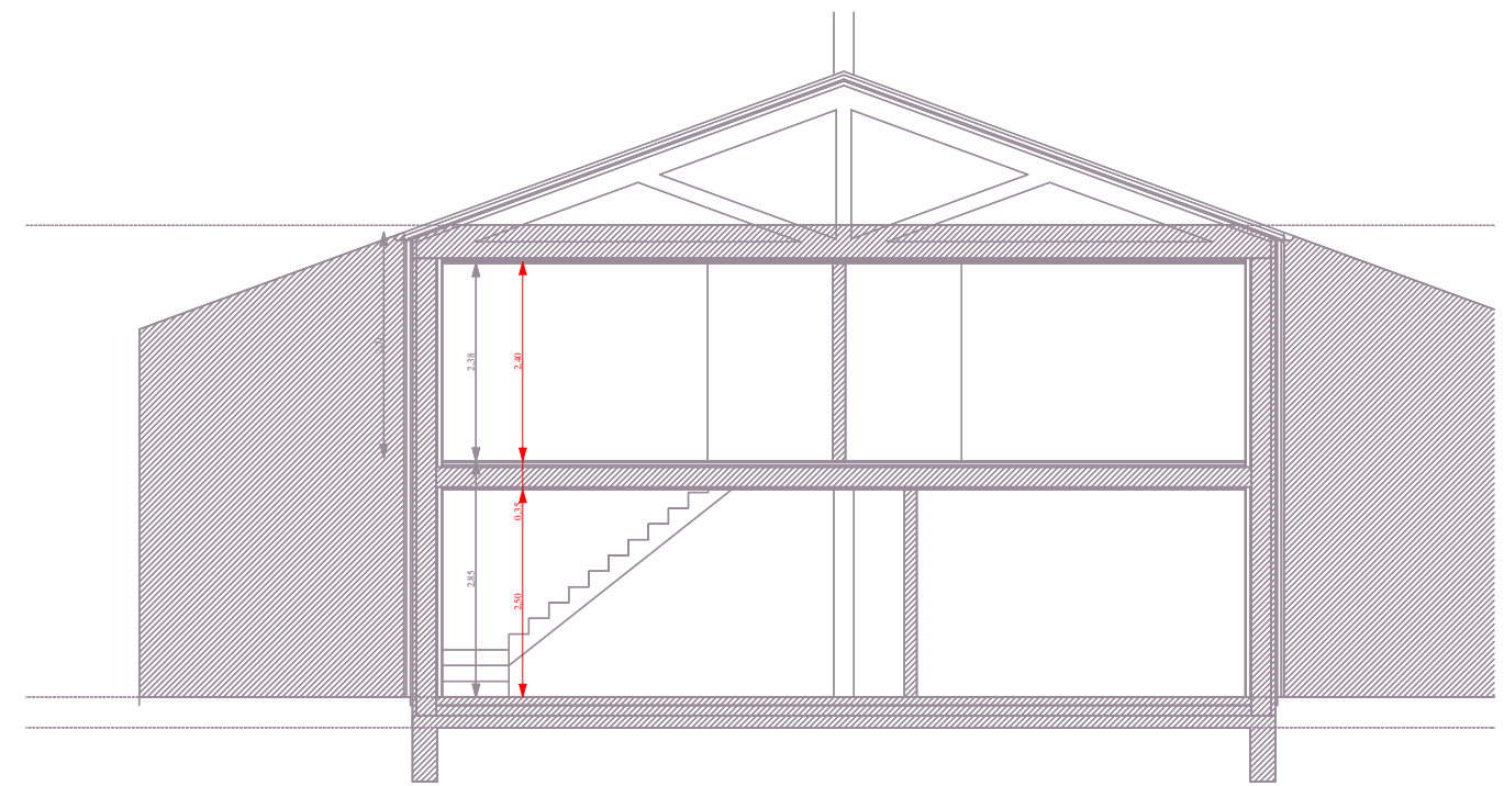
COUPE AA
