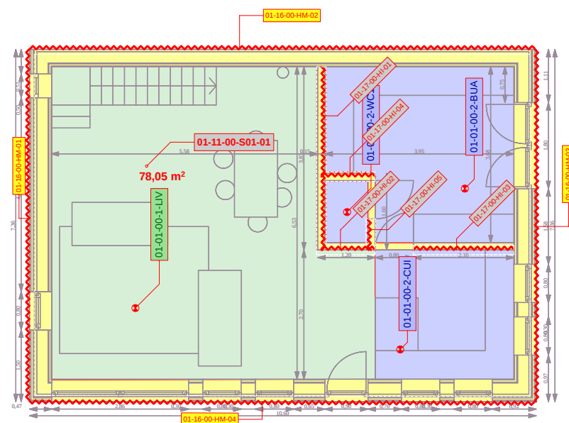
PLAN DU REZ DE CHAUSSEE
