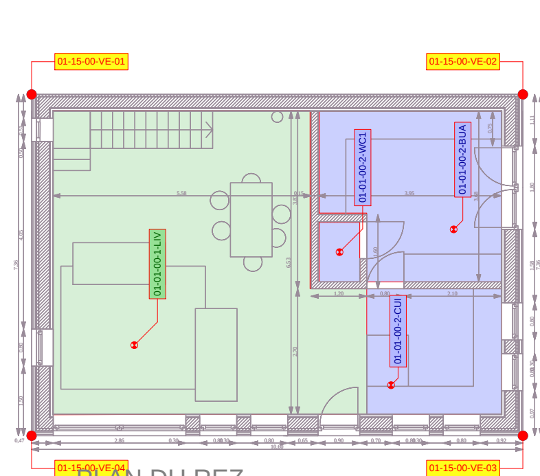
PLAN DU REZ DE CHAUSSEE
