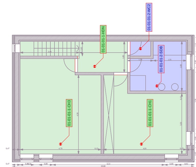
PLAN DU 1er ETAGE
